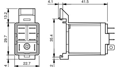
056.27 z przekaźnikiem
