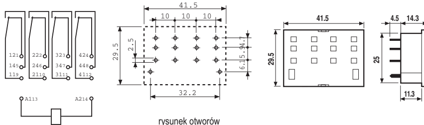
rysunek otworów montażowych 96.14
