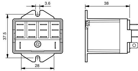
056.45 z przekaźnikiem
