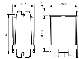
056.26 z przekaźnikiem
